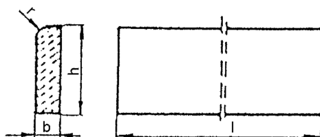
Rysunek 1. Kształt betonowego obrzeża chodnikowego Tabelica 1. Wymiary obrzeży
